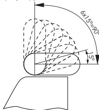
Схема положений регулируемых подголовников
